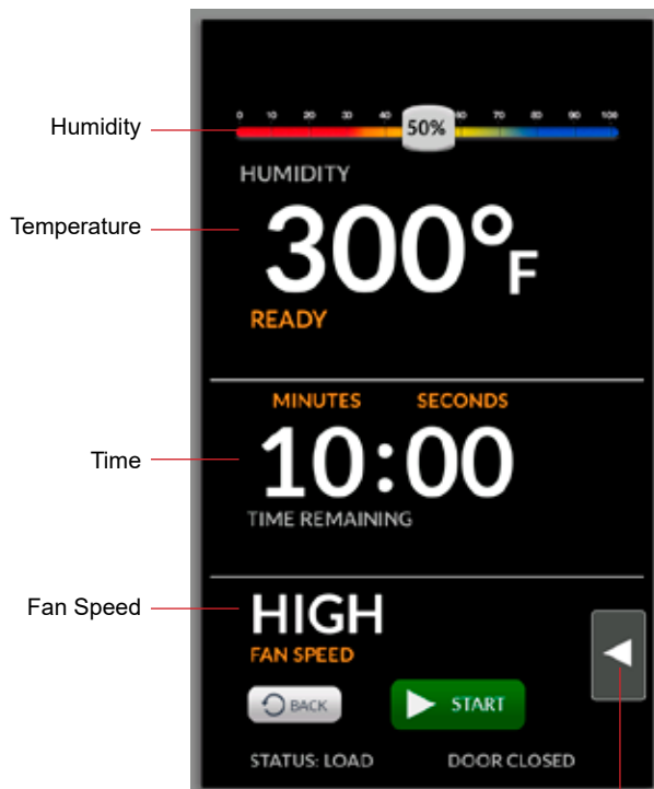
Flyout Menu
