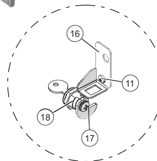
Optional Door Lock Parts
