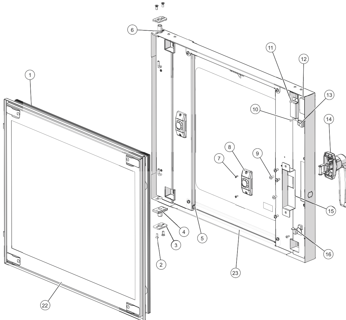
Optional Door Lock Parts
